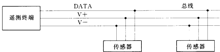
图 H.1 SDI 串行传感网络结构图
