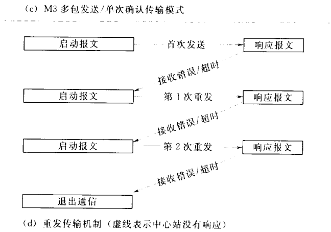
图 1 (二) 自报式报文传输链路示意图
