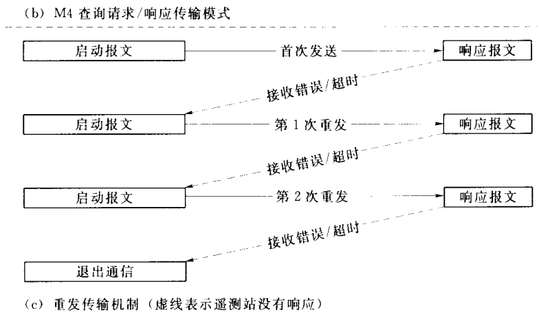
图 2 (二) 查询应答式报文传输链路示意图
