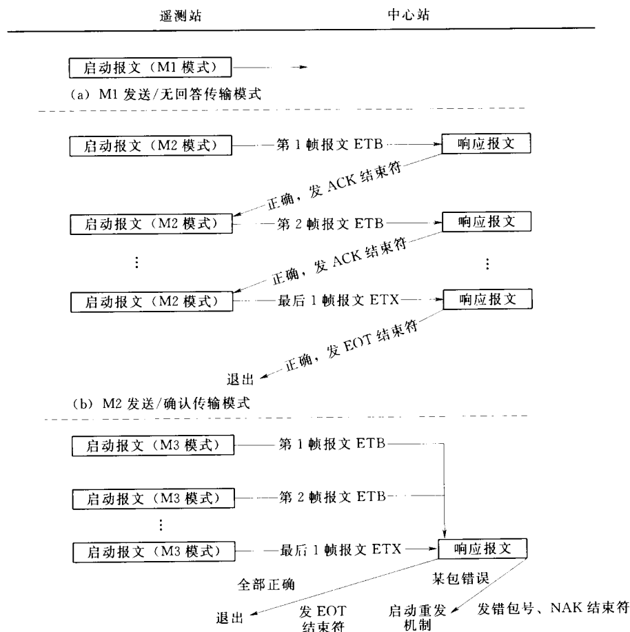
图 1 (一) 自报式报文传输链路示意图
