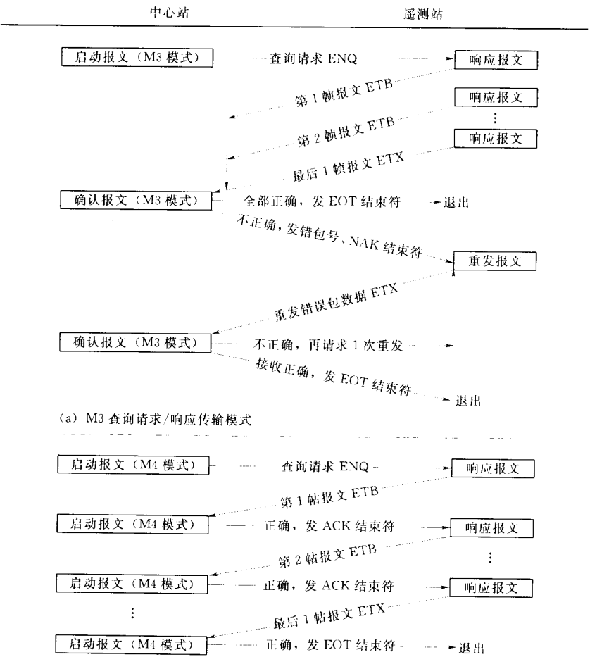
图 2 (一) 查询应答式报文传输链路示意图
